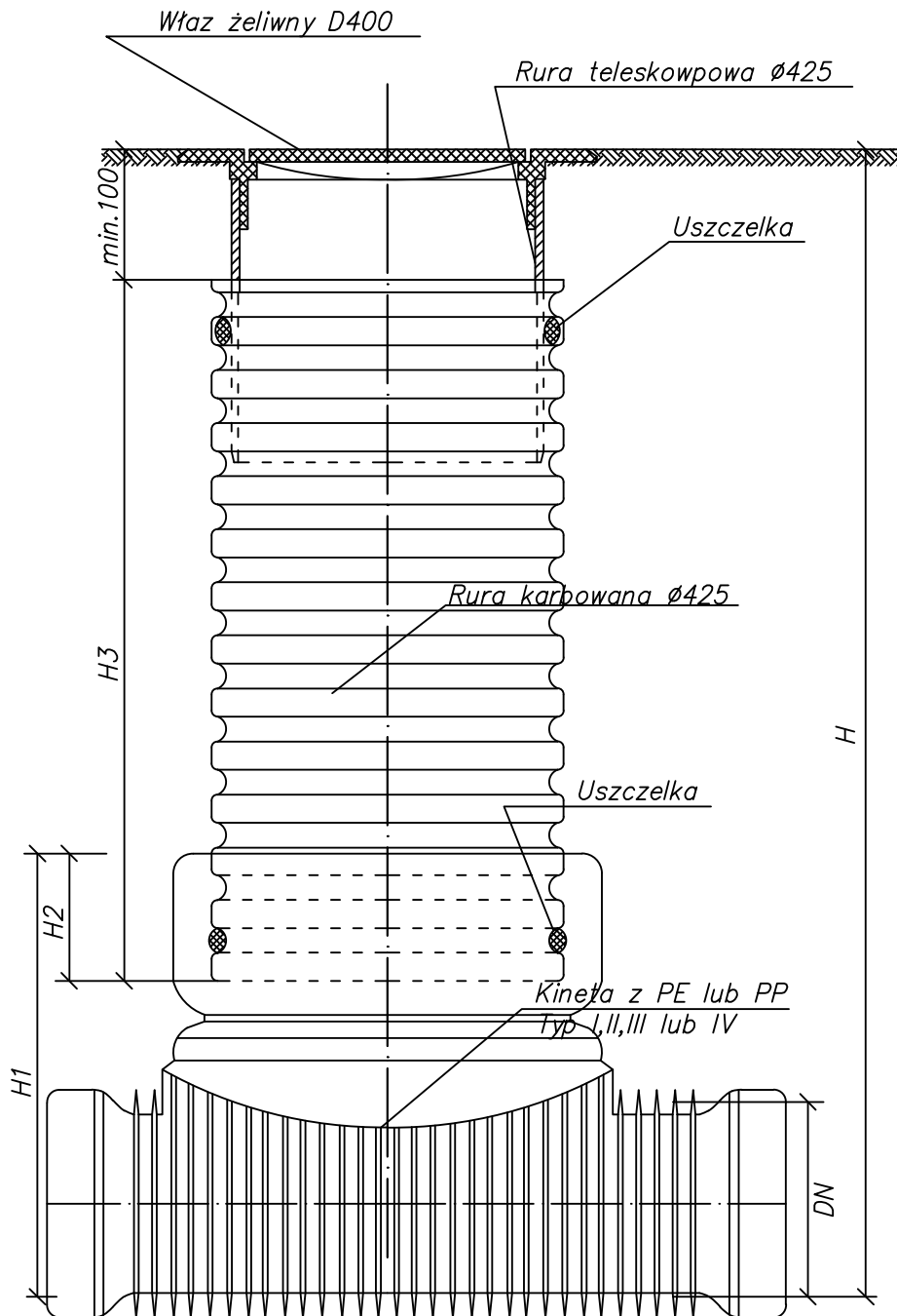
Studzienka kanalizacyjna \varnothing 425 niewłazowa
